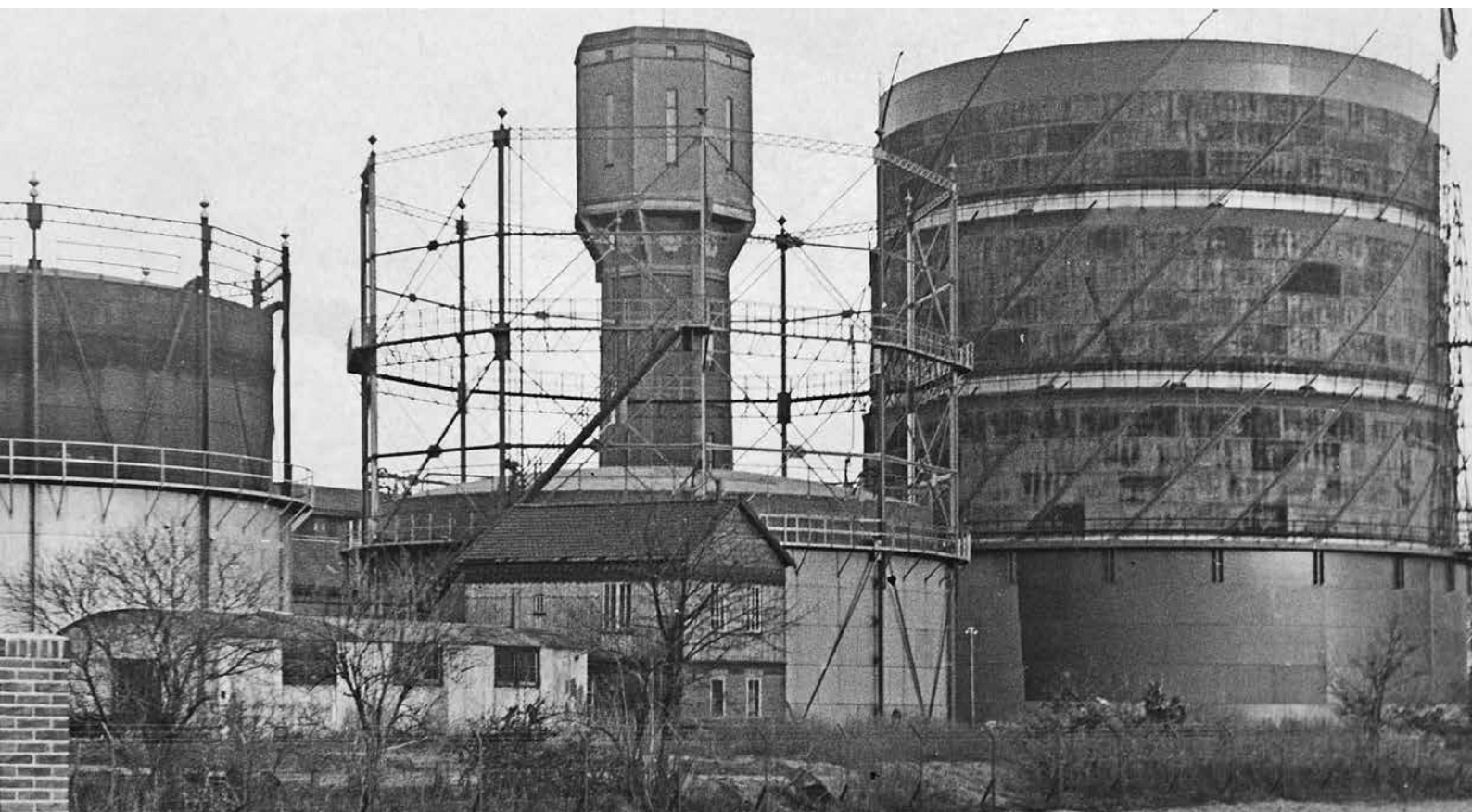
▲ De meest rechtse gashouder is de derde, die in 1933 geopend werd. De drie telescopische ringen zijn hier geheel uitgeschoven.
