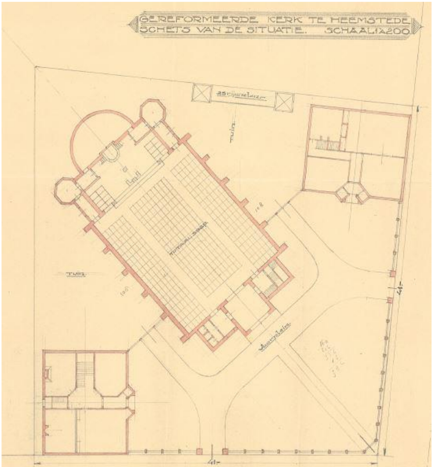
Schets uit 1918, gemaakt door de architecten Tijs de Bruin en Klaas Jonkheid. In het midden de kerk met links de pastorie en rechts de kosterij. Onderaan loopt de Koediefslaan, rechts de dan al geprojecteerde maar nog niet bestaande Van Slingelandtlaan.
